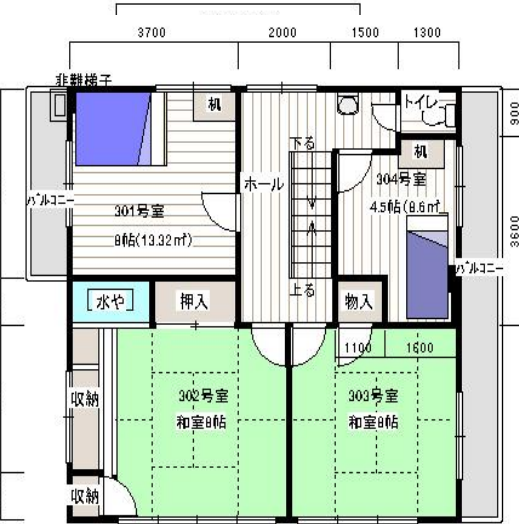
3階 平面図
